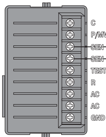
Блок питания
