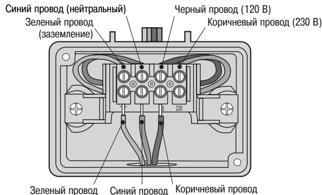
Рис. 2 – Распределительная коробка с клеммной колодкой (230 вольт)
