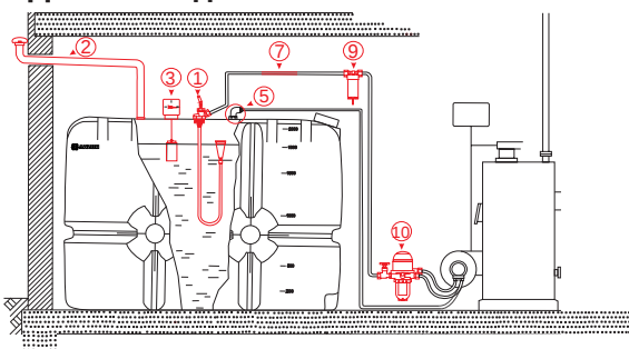
Для баков до 2 м³
