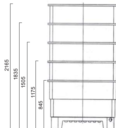
Штабелирование контейнеров КЛ500СП
