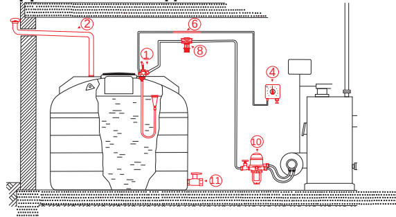
Для баков от 2 до 15 м³
